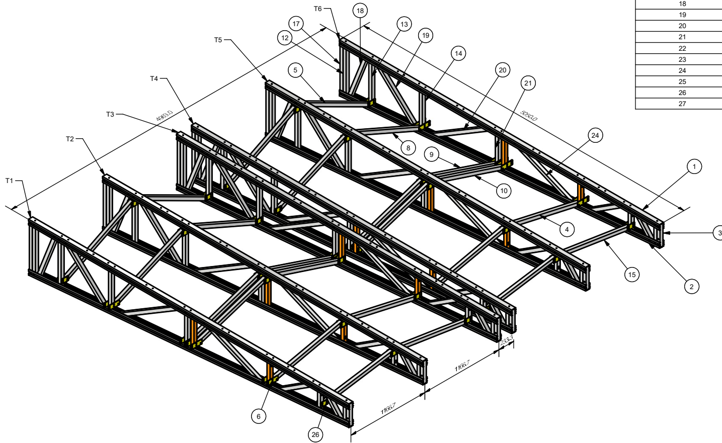
ISOMETRIC VIEW SCALE: 1 : 30
